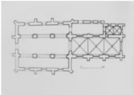
Rzut kaliskiego kościoła franciszkańskiego. Źródło: Architektura gotycka w Polsce , red. T. Mroczko, M. Arsyński, Warszawa 1995, t. 2, s. 412.
